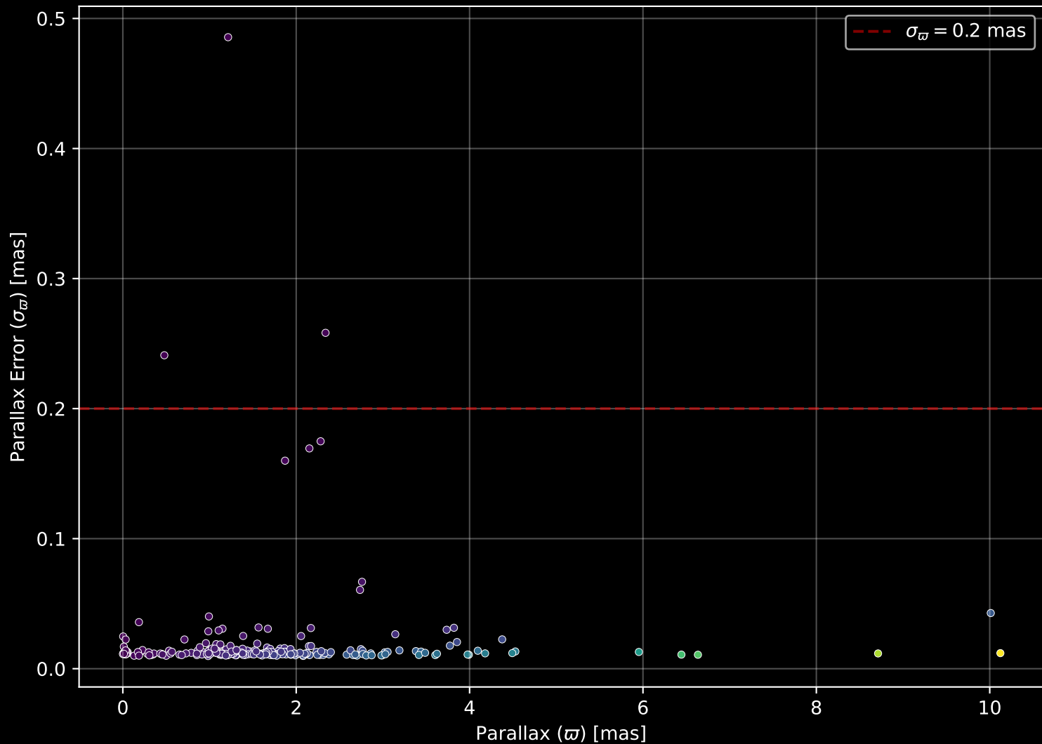
GALAH DR4 Field: [92] Parallax Quality (n= 241)
