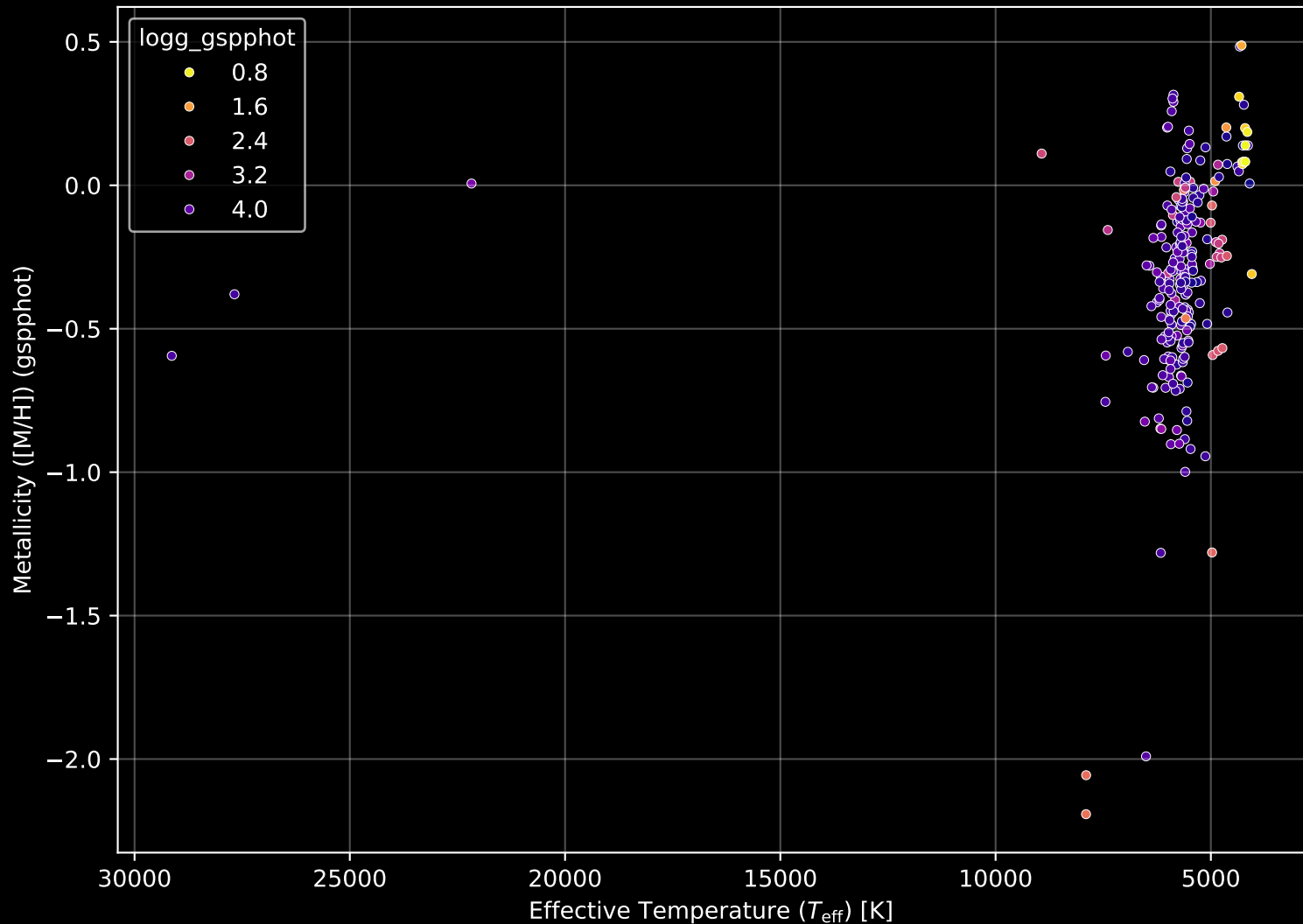
GALAH DR4 Field: [92] Stellar Population Parameters (n= 241)
