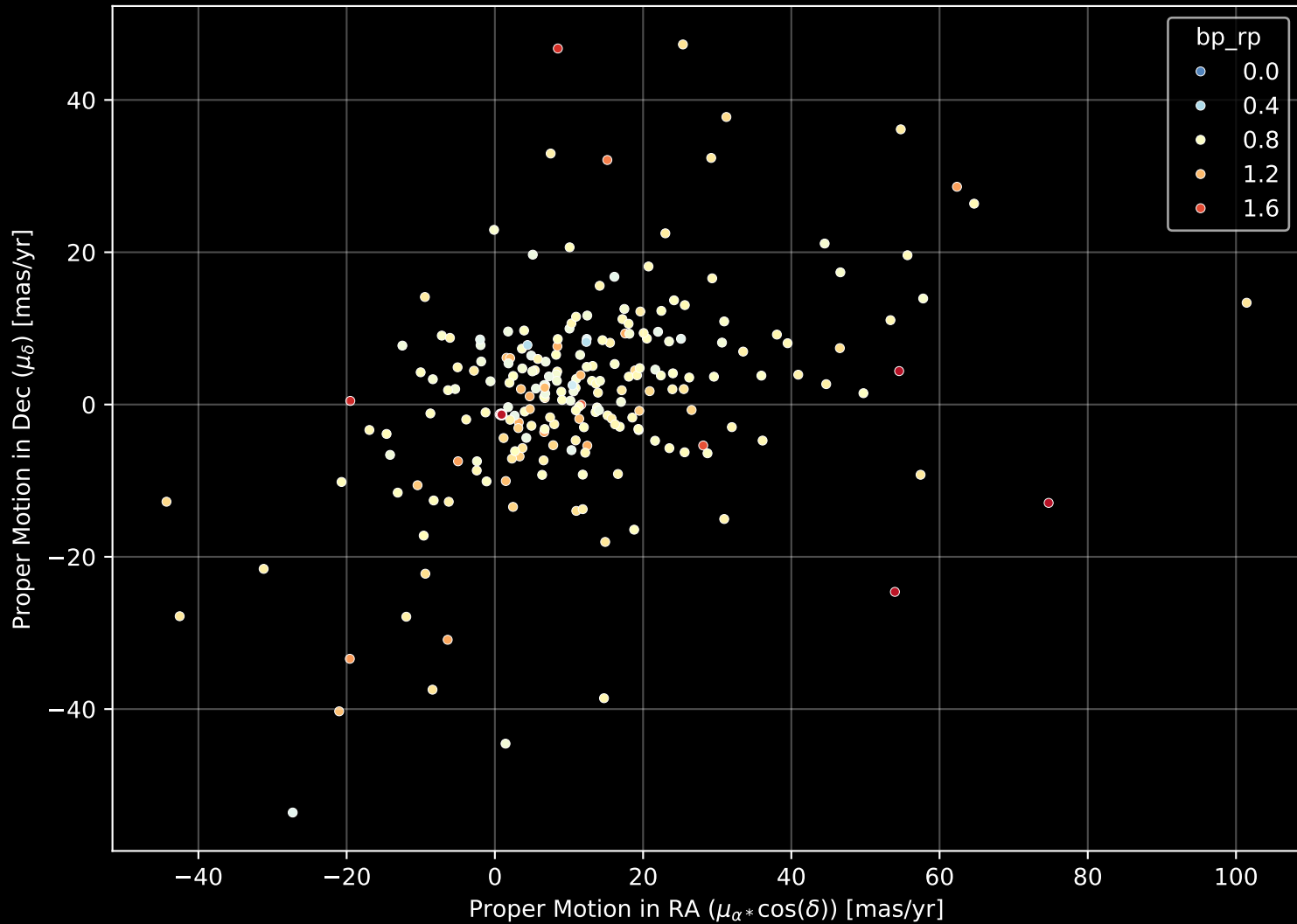
GALAH DR4 Field: [92] Proper Motion Diagram (n= 241)
