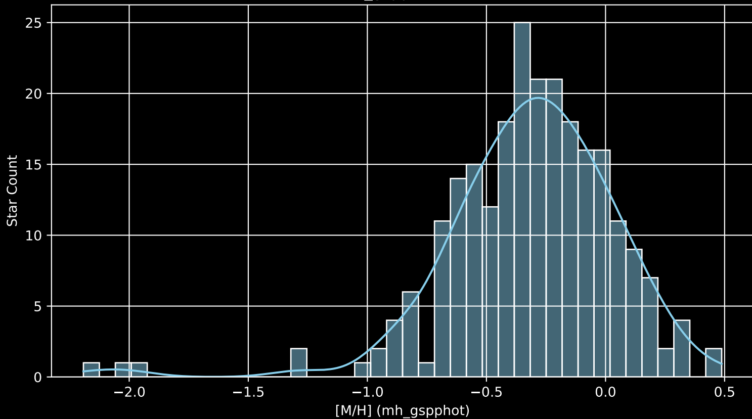
GALAH DR4 Field: [92] [M/H] (mh_gspphot) (n= 241)
