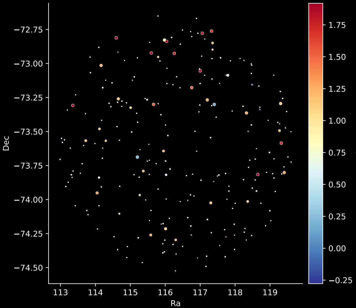
GALAH DR4 Field: [92] Stars: 241
